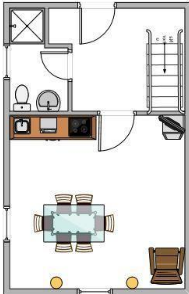
Přízemí
